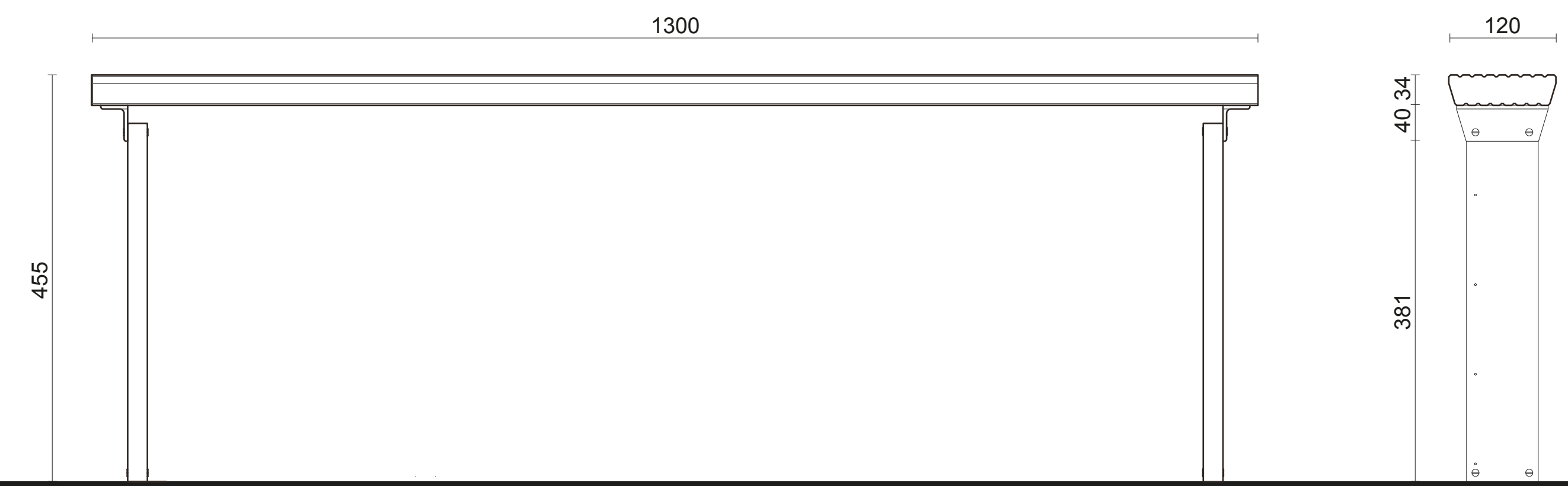
LAVIČKA KE KRÁTKÉMU POSEZENÍ, nejmenší verze, pohled čelní M 1:5, pohled boční M 1:5
