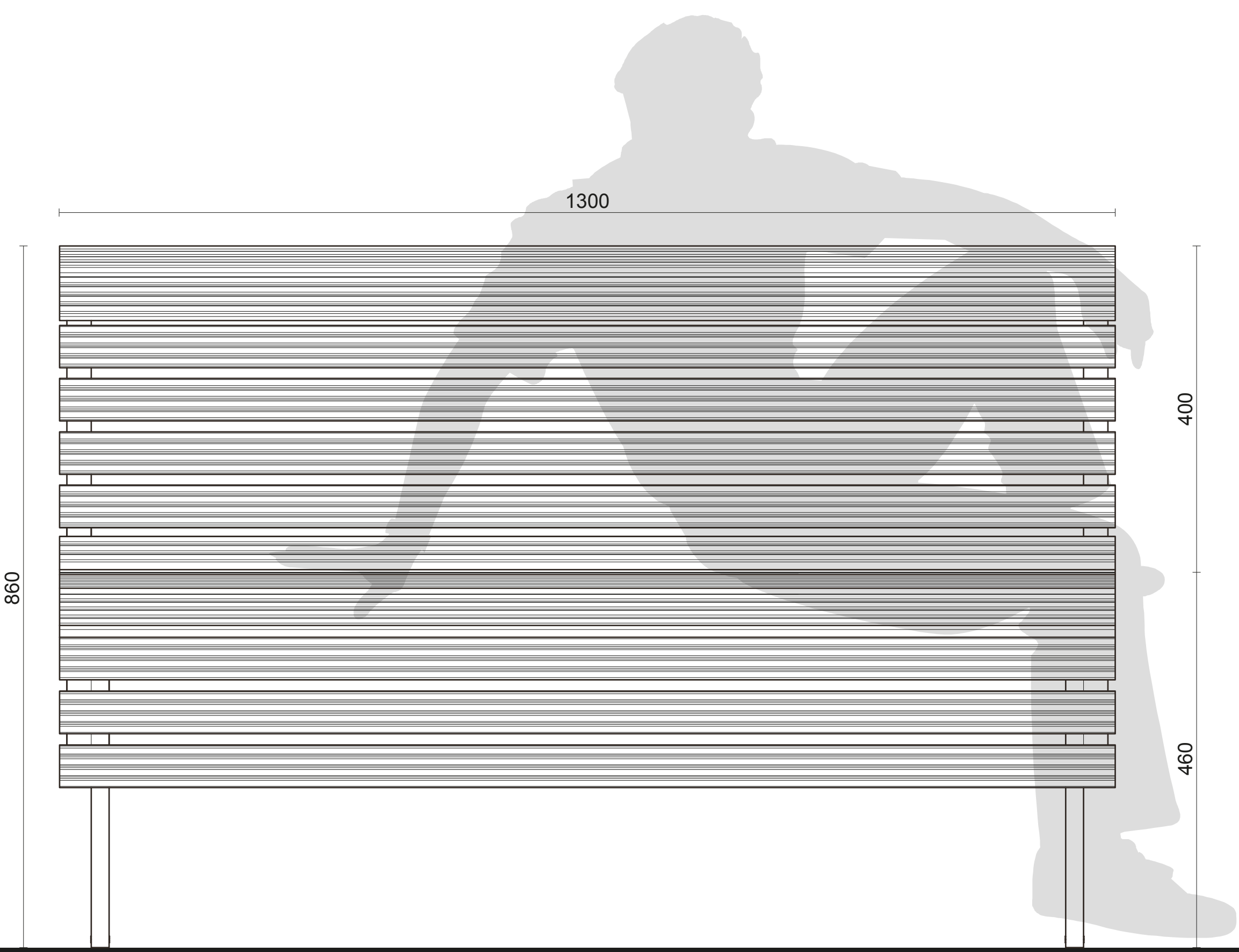
LAVIČKA K DLOUHÉMU POSEZENÍ, klasická verze, pohled čelní M 1:5, pohled boční M 1:5
