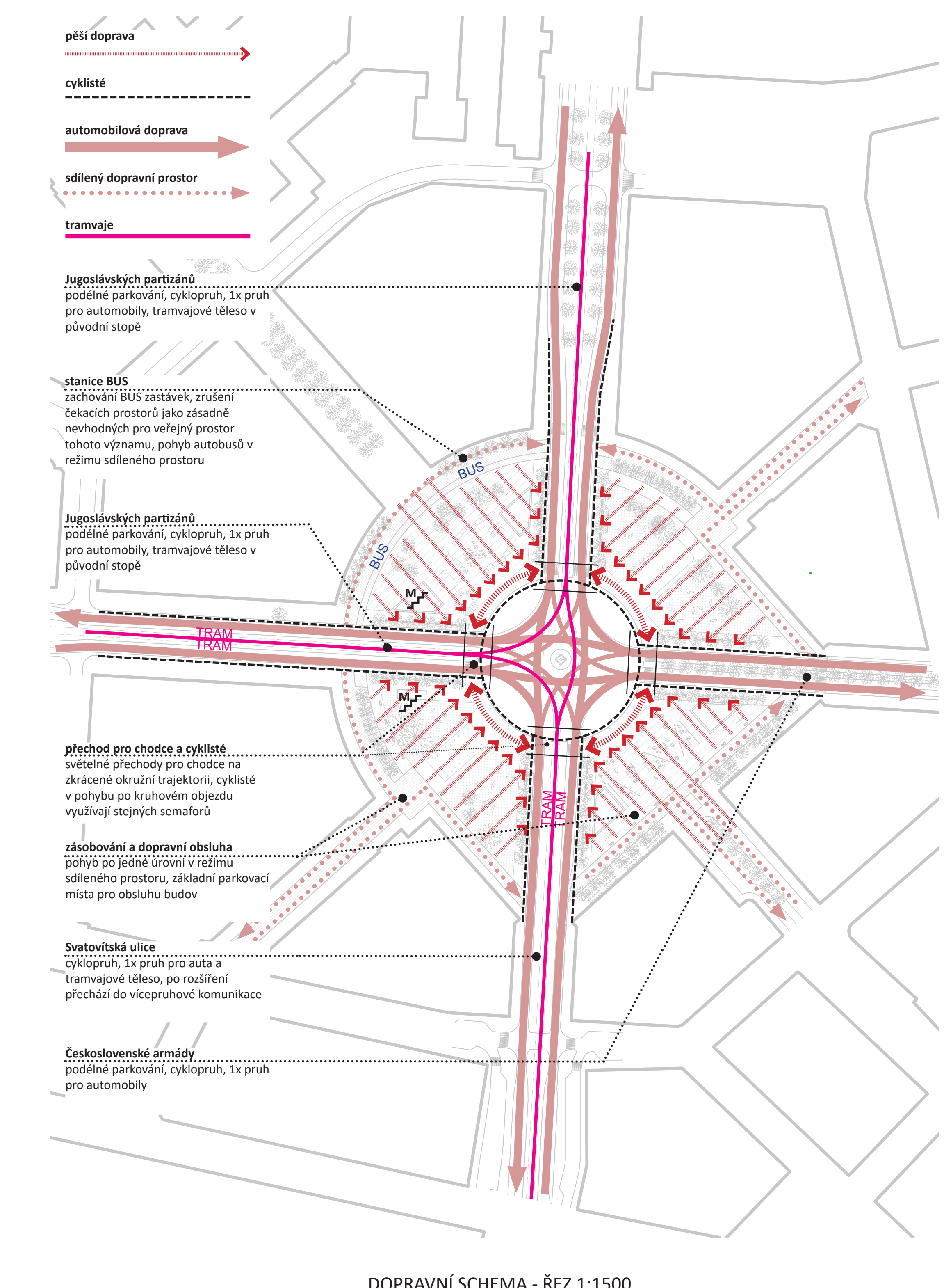
DOPRAVNÍ SCHEMA - ŘEZ 1:1500
