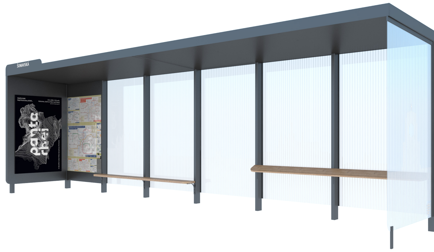
2. prodloužený půdorysný rozměr plně bočnice, vybavení přístřešku minimální
