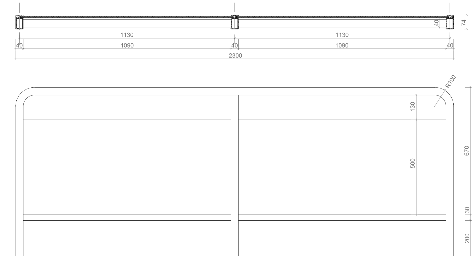
ZÁBRADLÍ S VÝPLNÍ, 1:10
