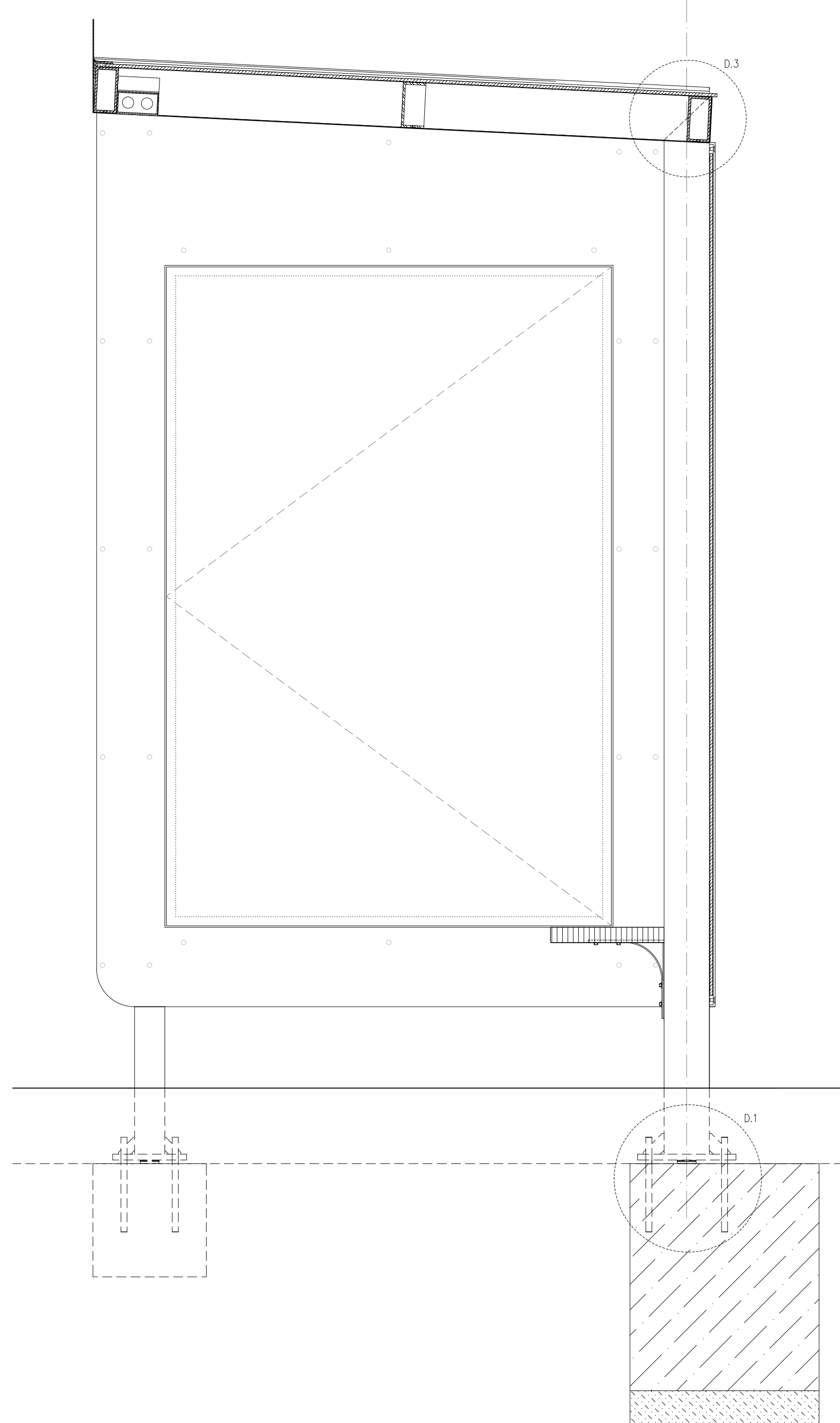
PŘÍČNÝ REZ, 1:10
