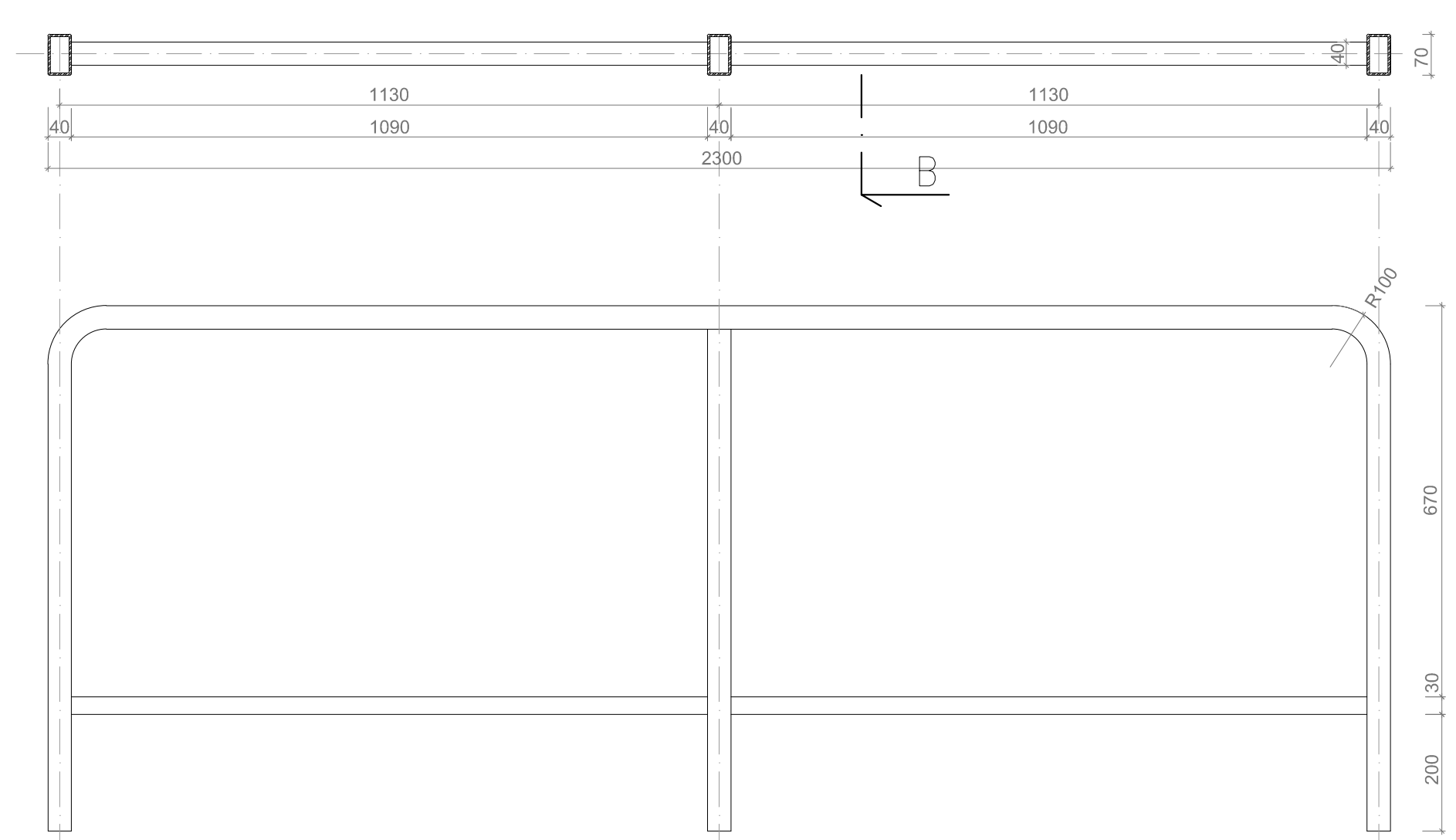
ZÁBRADLÍ S VÝPLNÍ, 1:10
