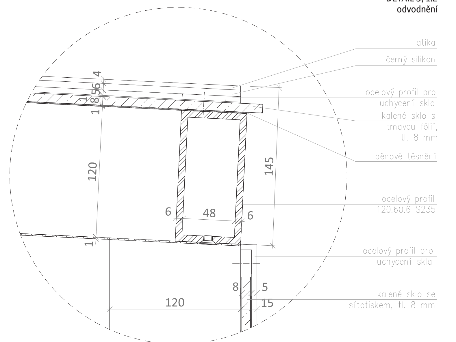
DETAIL 3, 1:2 odvodnění
