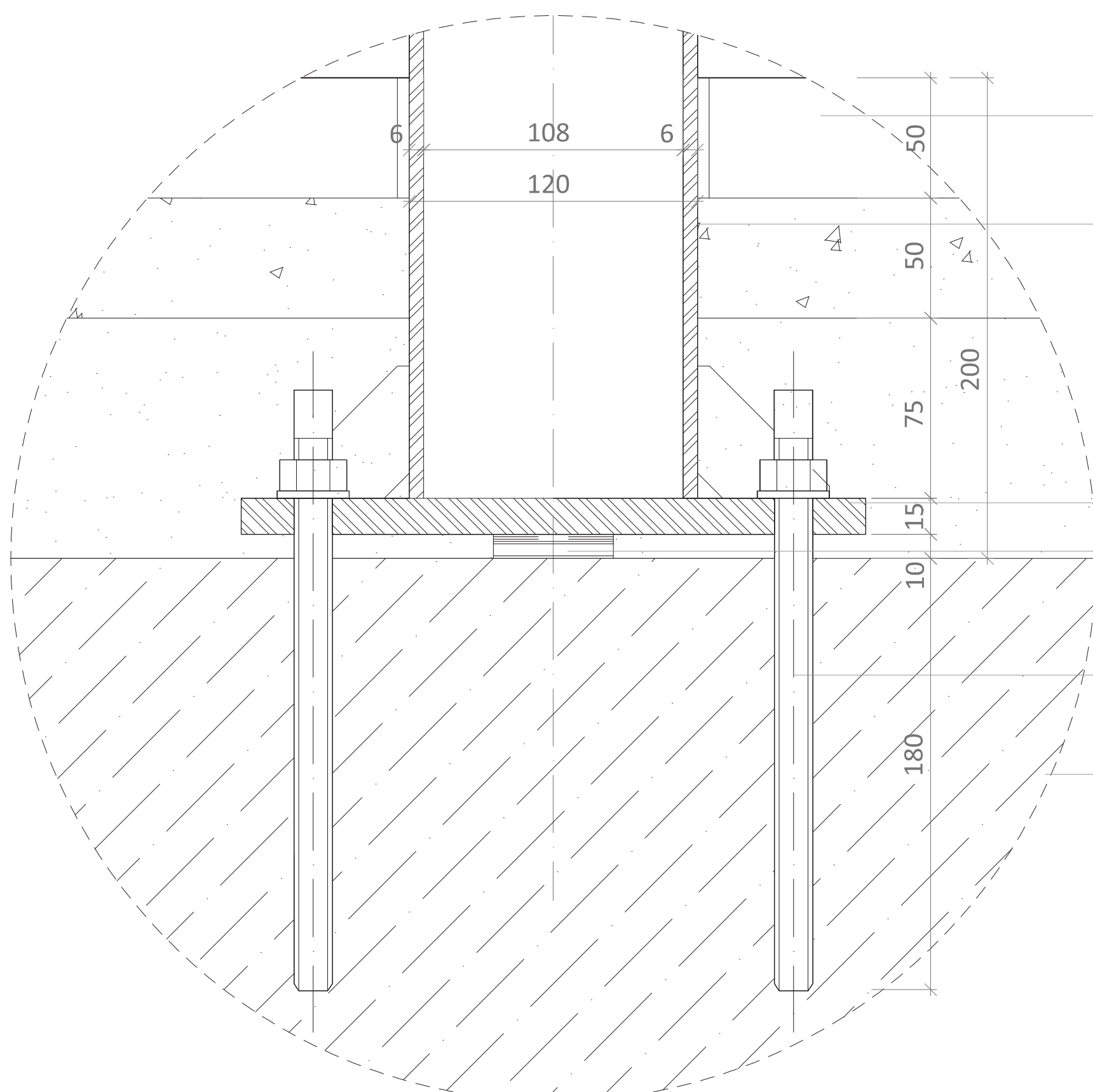
DETAIL 1, 1:2 kotvení základů
