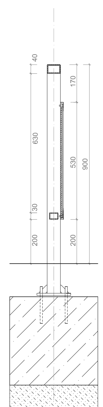
REZ ZÁBRADLÍM, 1:10
