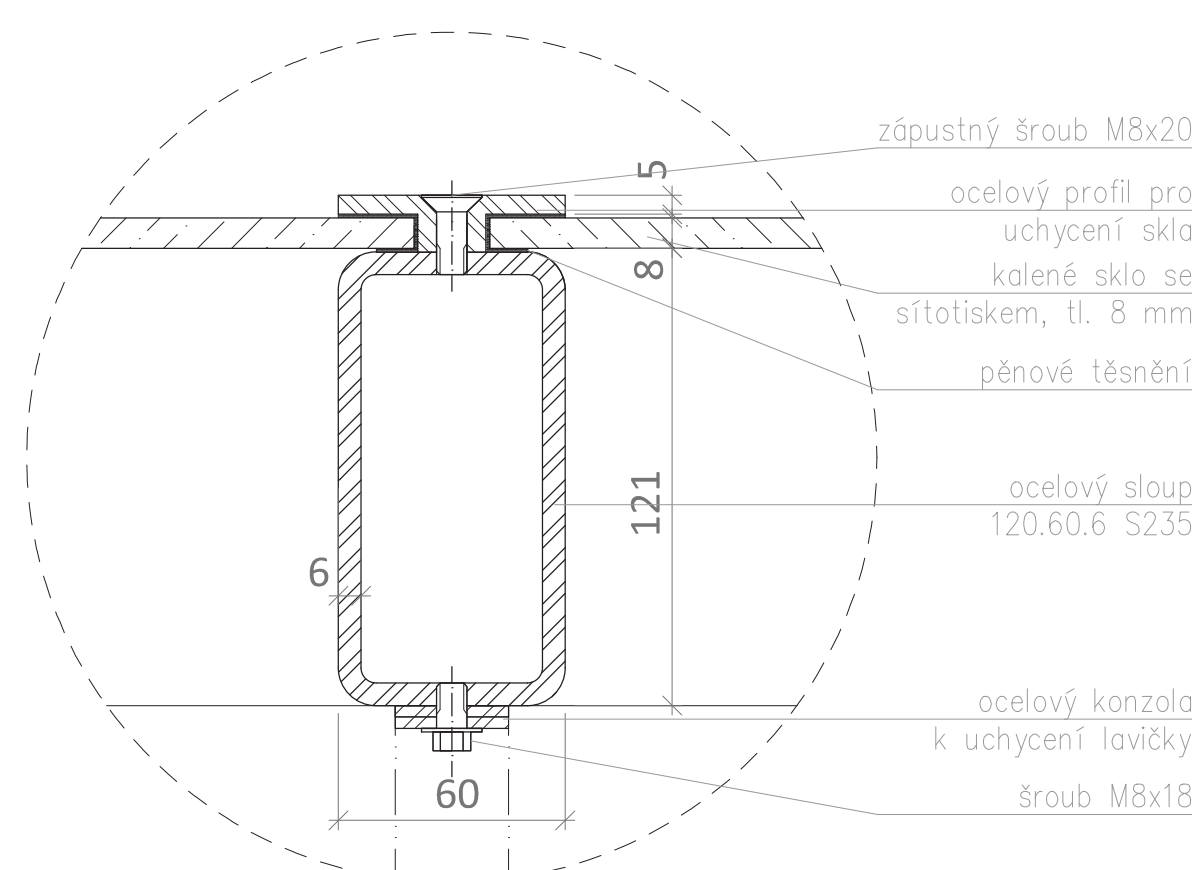
DETAIL 2, 1:2 ukotvení skleněných výplní
