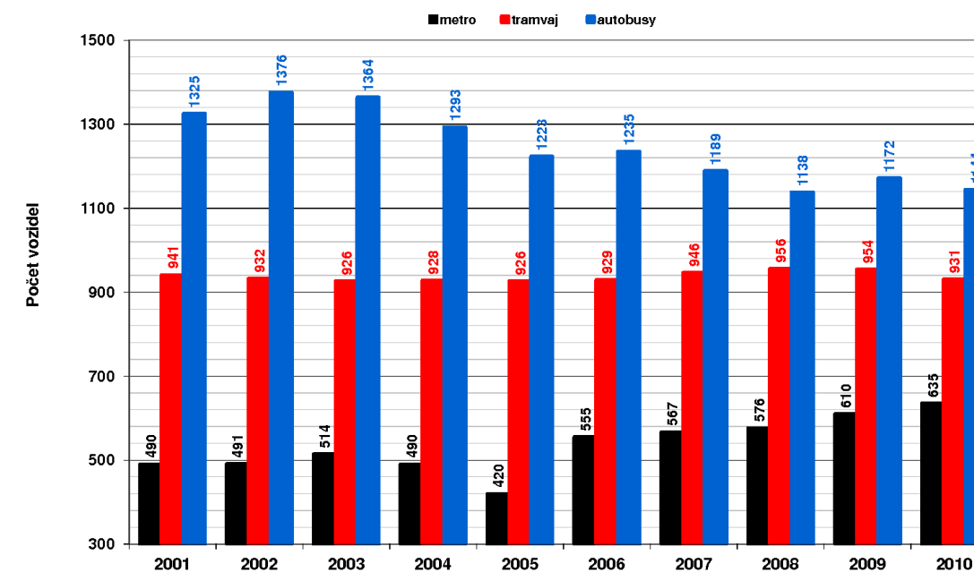
Graf Provozní stav vozového parku prostředků veřejné dopravy
