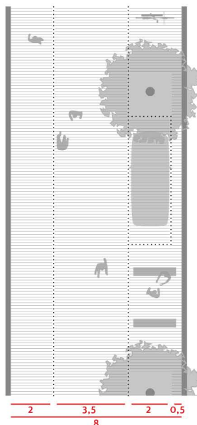
s07 LOKÁLNÍ ULICE (ŠÍŘKA 8 M) Lokální ulice se sdíleným prostorem pro všechny uživatele v jedné úrovni.
